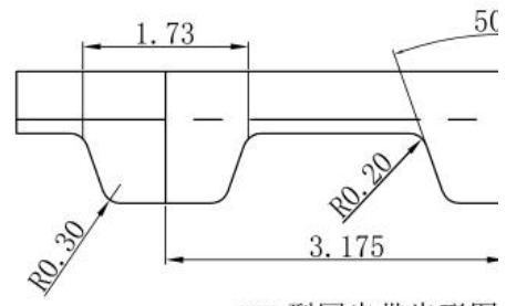
XXL型同步带齿形图
