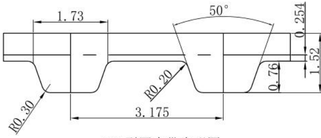
XXL型同步带齿形图
