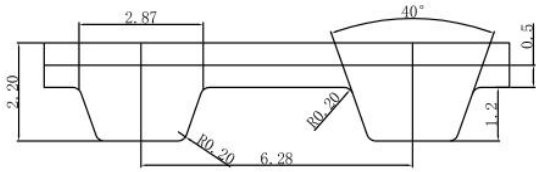
2m同步带齿形图
