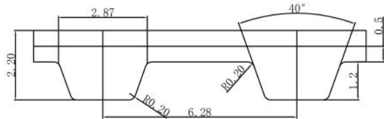
2m同步带齿形图
