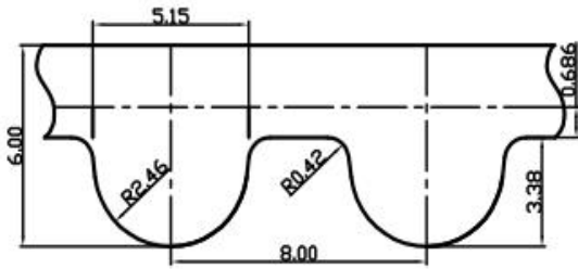
8M带齿形图
