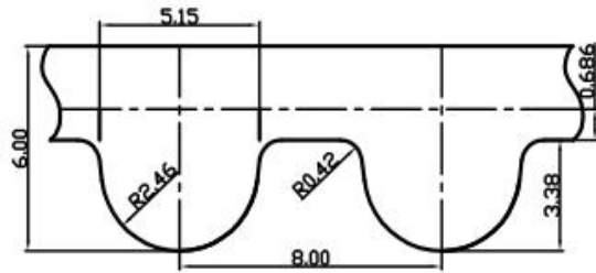
8M带齿形图
