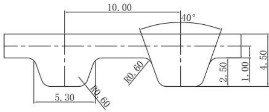
T10型同步带齿形图
