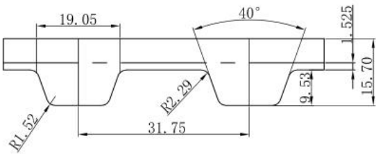
XXH型同步带齿形图
