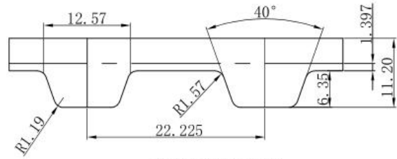
XH型同步带齿形图
