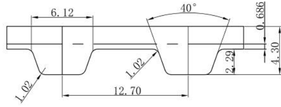
H型同步带齿形图
