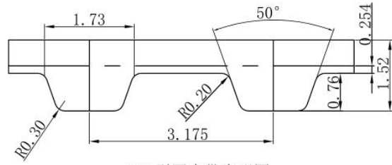
XXL型同步带齿形图
