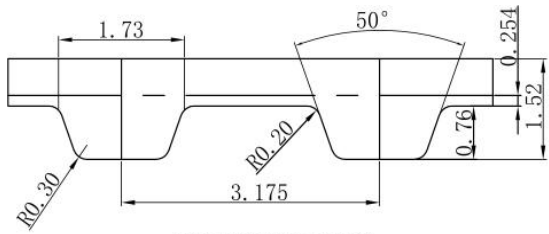
XXL型同步带齿形图
