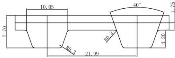
7m同步带齿形图
