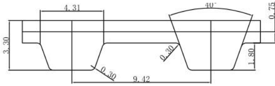
3m同步带齿形图
